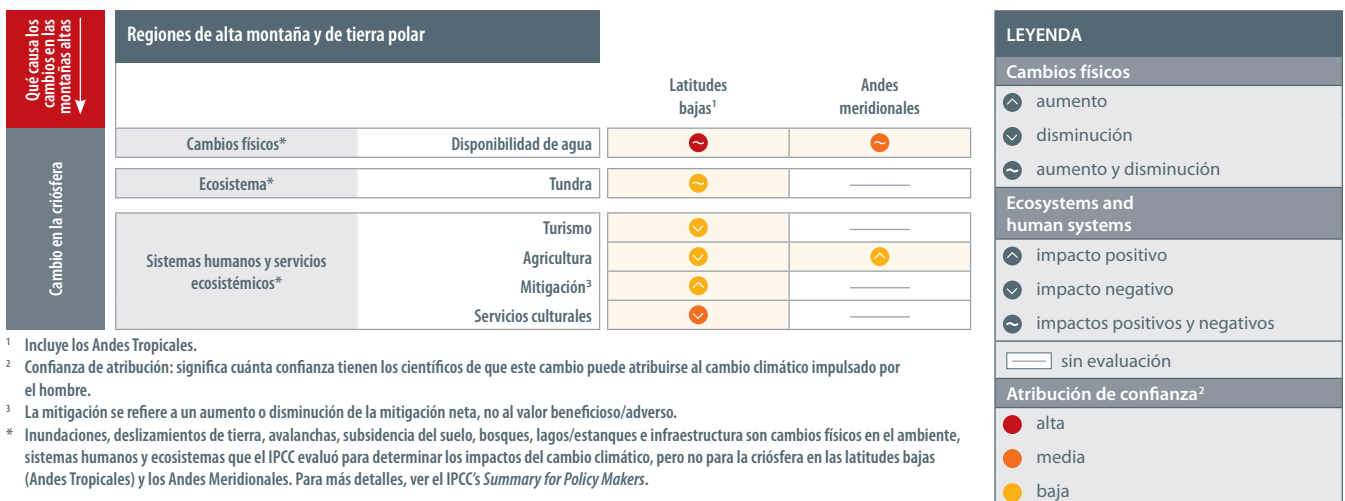
Figura 4: Cómo los cambios en la atmósfera y el clima han afectado a la criósfera 60
