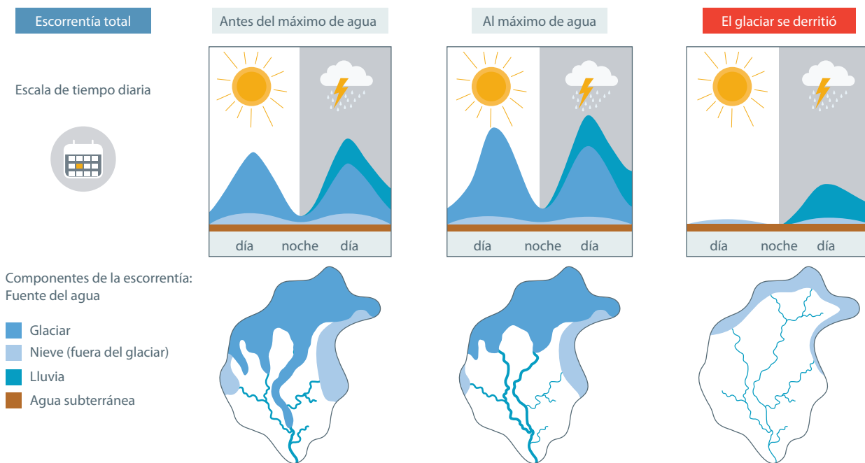
Figura 5: Una imagen simplificada de cómo cambia la escorrentía en una cuenca cuando un glaciar se derrite 62
