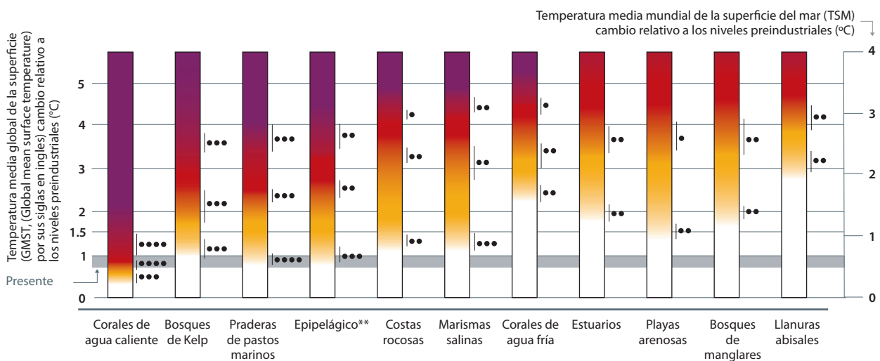
Figura 2: Cada grado de calentamiento global afectará aún más los ecosistemas costeros 20
