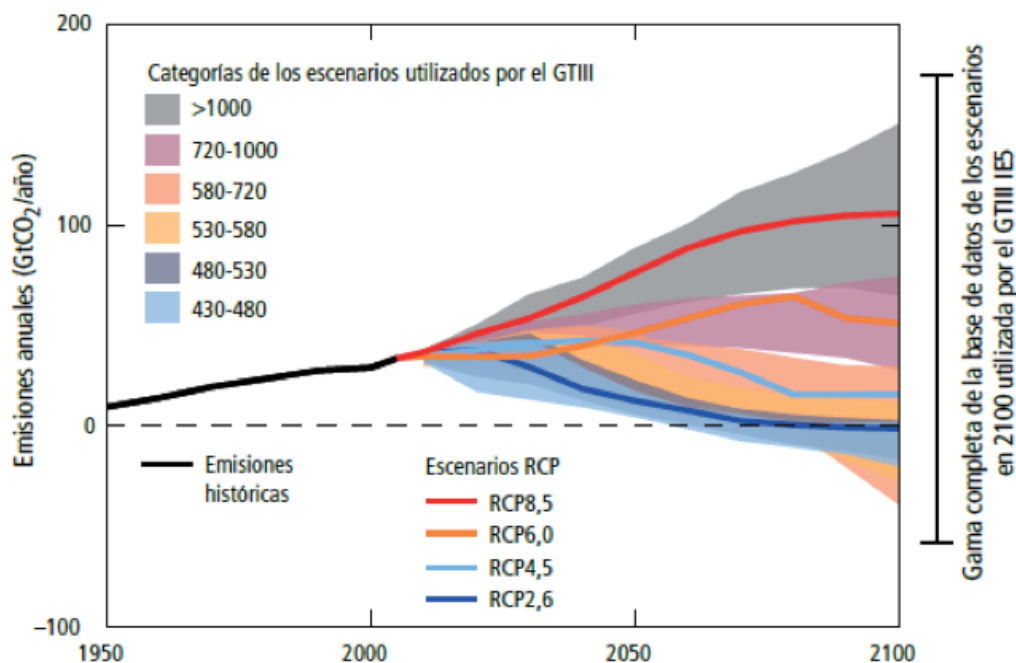
Figura 4: Emisiones Antropógenas de CO 2 anuales
