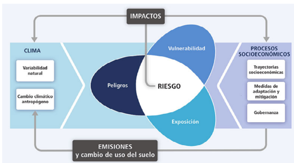
Figura 5: Esquema de riesgo de los impactos conexos al clima.
