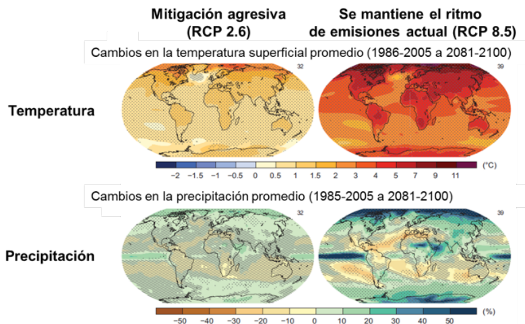
Figura 5: Cambios promedio proyectados en la temperatura de la superficie terrestre y la precipitación
