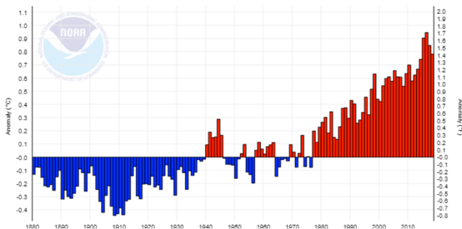
Figura 2: Anomalías de la temperatura de la tierra a nivel global
